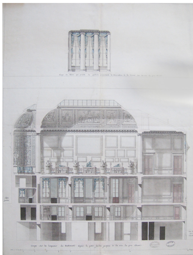
fig. 3 : J-A Raymond, Hôtel Lebrun, coupe de la galerie d'exposition. Paris, Archives Nationales, Z1J 1314 (28) pièce 1. (cl. de l'auteur).
