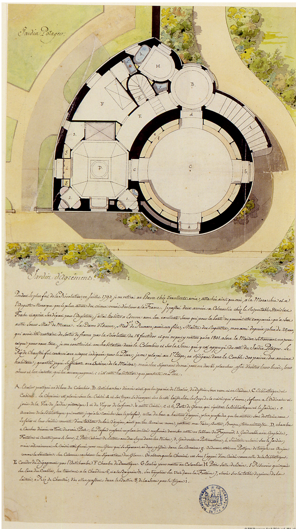
fig. 6 : Pierre-Adrien Pâris, Plan du colombier d'Escures, BMB vol. 484 n° 45. © BM Besançon.
